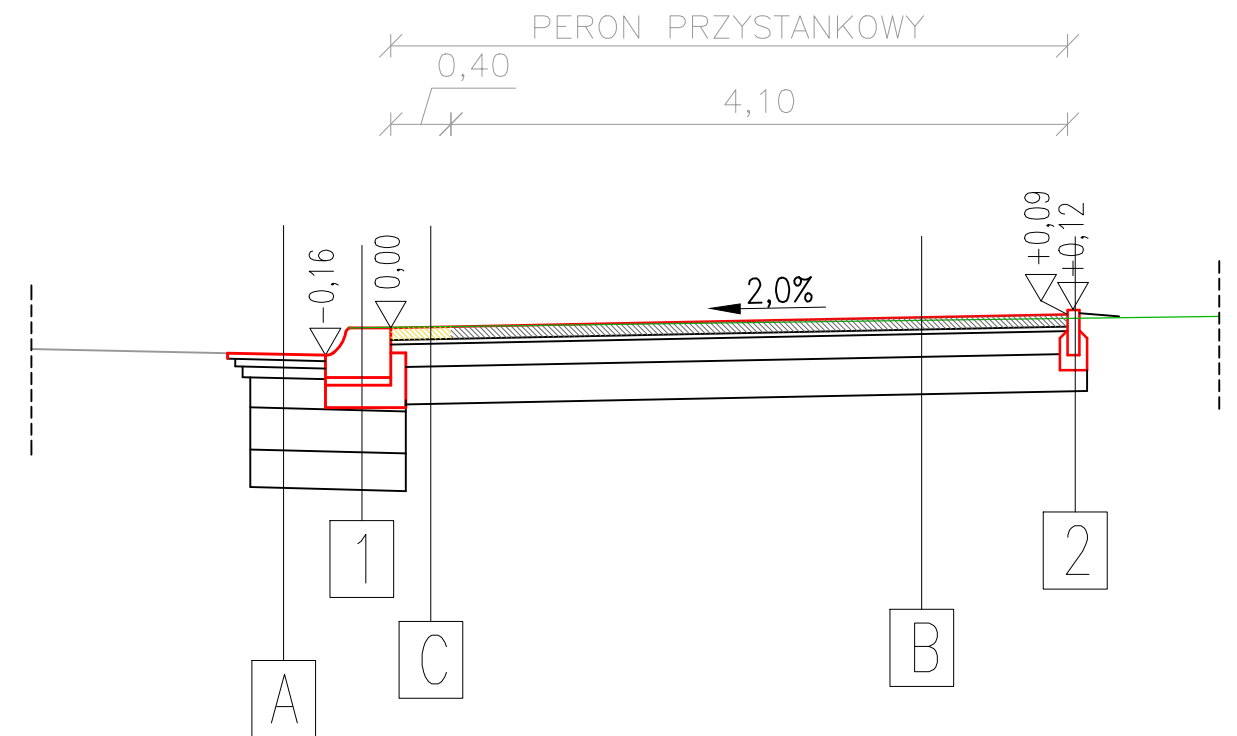
Przekrój peron
