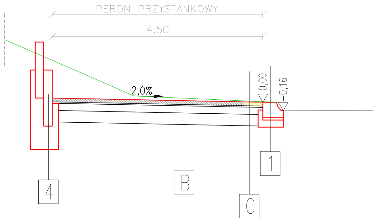
Przekrój peron
